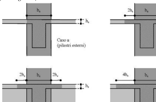
Fig. 7.4.1 – Larghezza collaborante delle travi
