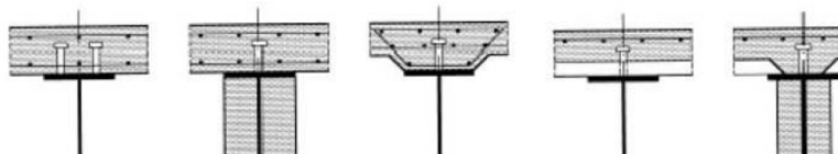
Fig. 4.3.3 -Tipologie di sezione composte per travi
