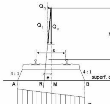
Fig. 5.2.5 - Distribuzione trasversale in rettilineo delle azioni per mezzo delle traverse e del ballast. In figura, Q_n rappresenta la forza centrifuga definita al successivo §5.2.2.3.1
