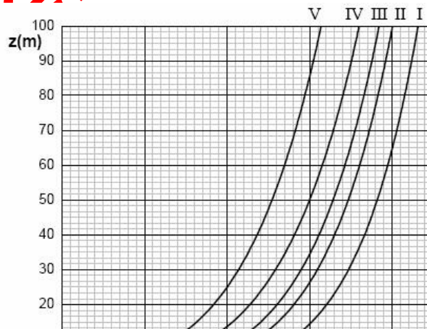
Fig. 3.3.3 - Andamento del coefficiente di esposizione ce in funzione dell'altezza sul suolo (per c_t = 1 )
