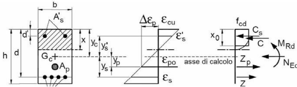
Fig. 4.1.4 – Sezione pressoinflessa
