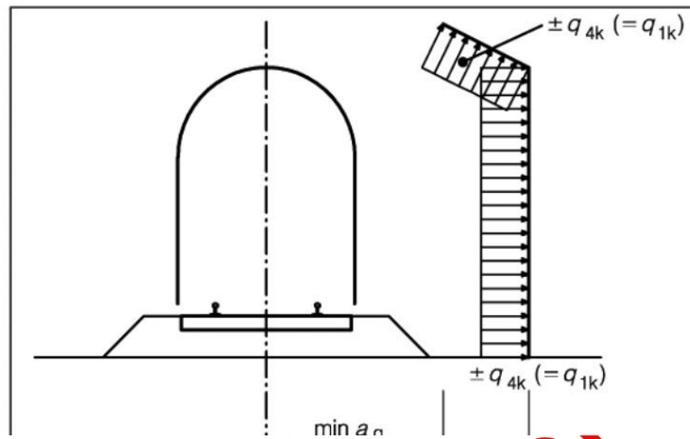
Fig. 5.2.11 - Definizione della distanza \max a_g e \min a_g dall'asse del binario
