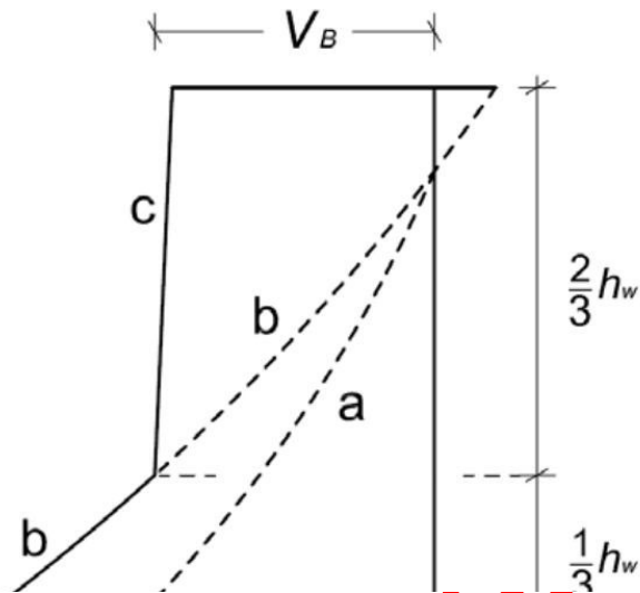
Fig. 7.4.5 – Diagramma di involuppo delle forze di taglio nelle pareti di strutture miste
