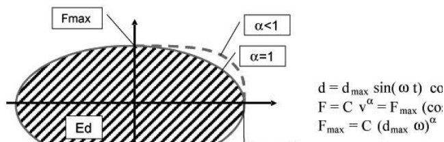
Fig. 11.9.2 – Dispositivi a comportamento viscoso
