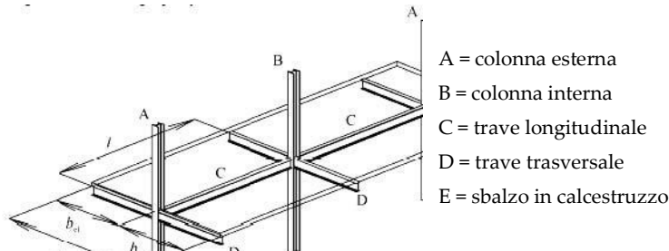
Fig. 7.6.2 - Definizione degli elementi in una struttura intelaiata
