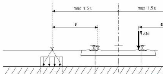
Fig. 5.2.12 - Caso 1
