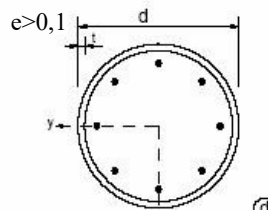
Figura 4.3.7 - Sezione tipo di colonna composta circolare riempita di calcestruzzo in cui è possibile considerare il confinamento del calcestruzzo
