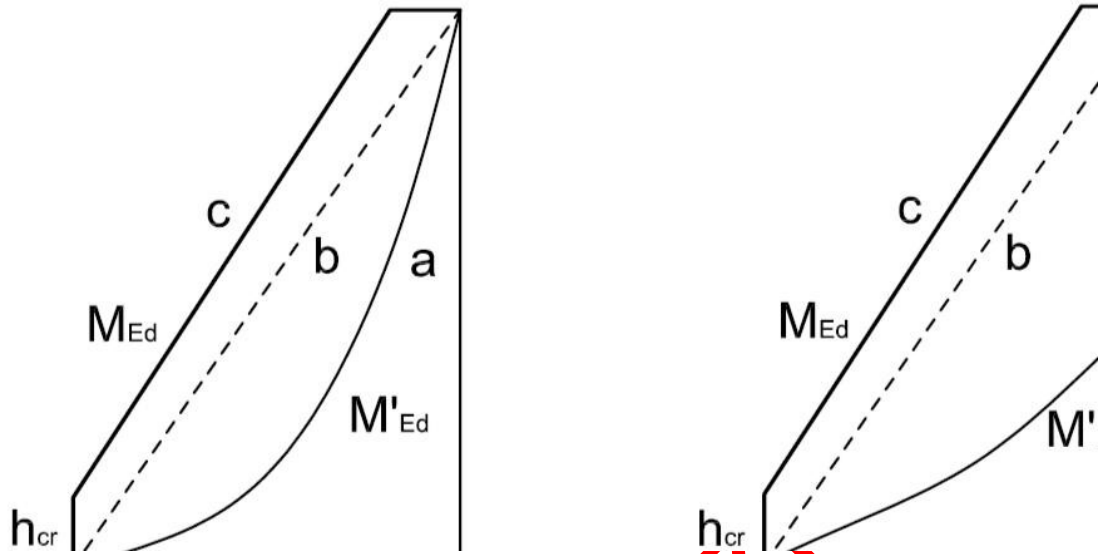
Fig. 7.4.4 – Traslazione del diagramma dei momenti flettenti per strutture a pareti e strutture miste
