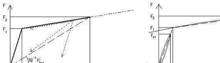
Fig. 11.9.1 - Diagrammi forza - spostamento per dispositivi non lineari
