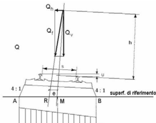
Fig. 5.2.6 - Distribuzione trasversale in curva delle azioni per mezzo delle traverse e del ballast. In figura, Q_h rappresenta la forza centrifuga definita al successivo §5.2.2.3.1
