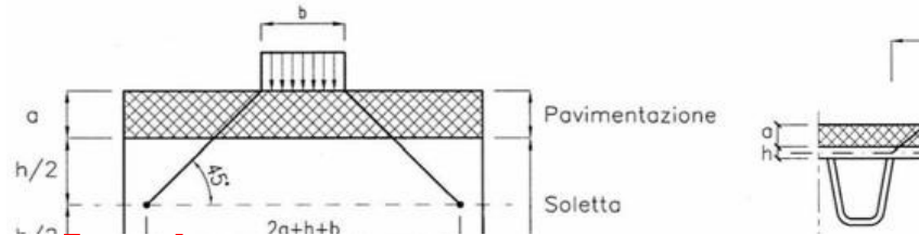
Fig. 5.1.3a - Diffusione dei carichi concentrati nelle solette
