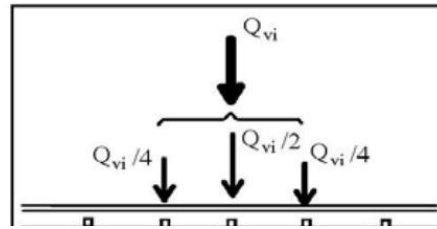
Fig. 5.2.3 - Distribuzione longitudinale dei carichi assiali
