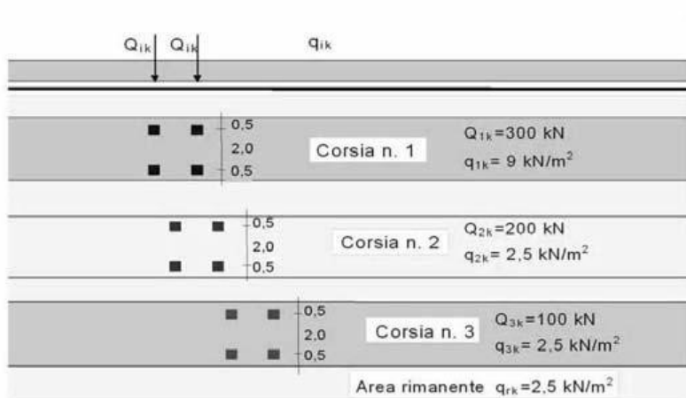
Schema di carico 1 (dimensioni in [m])
