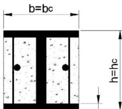
Fig. 7.6.1 - Rapporti dimensionali
