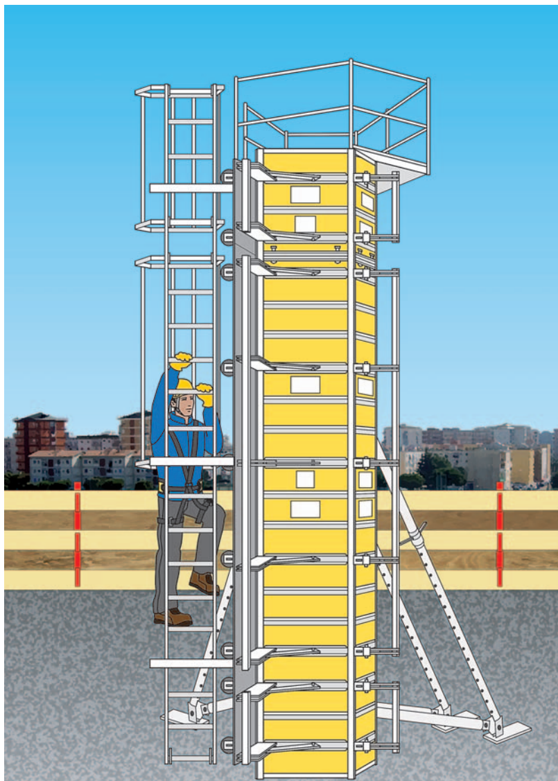
Figura 3 - Cassaforma verticale prefabbricata a telaio per pilastri
