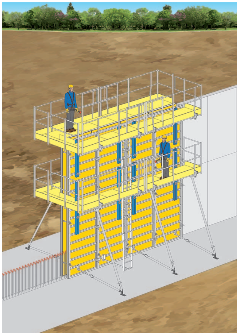
Figura 5 - Cassaforma verticale prefabbricata a telaio
